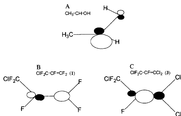
Fig. 1. Natural frontier orbitals: A SOMO, B LUMO, C LUMO.
